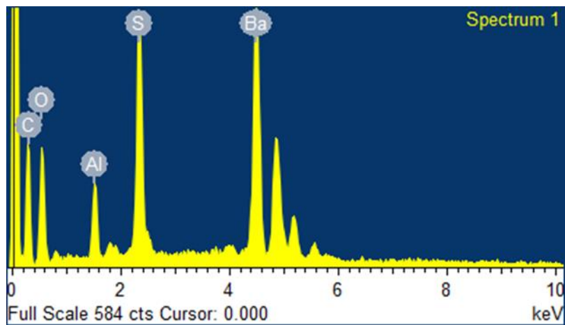
Figura 9. SEM de muestra
