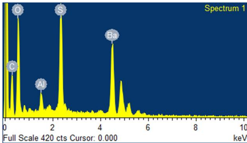
Figura 11. SEM de muestra
