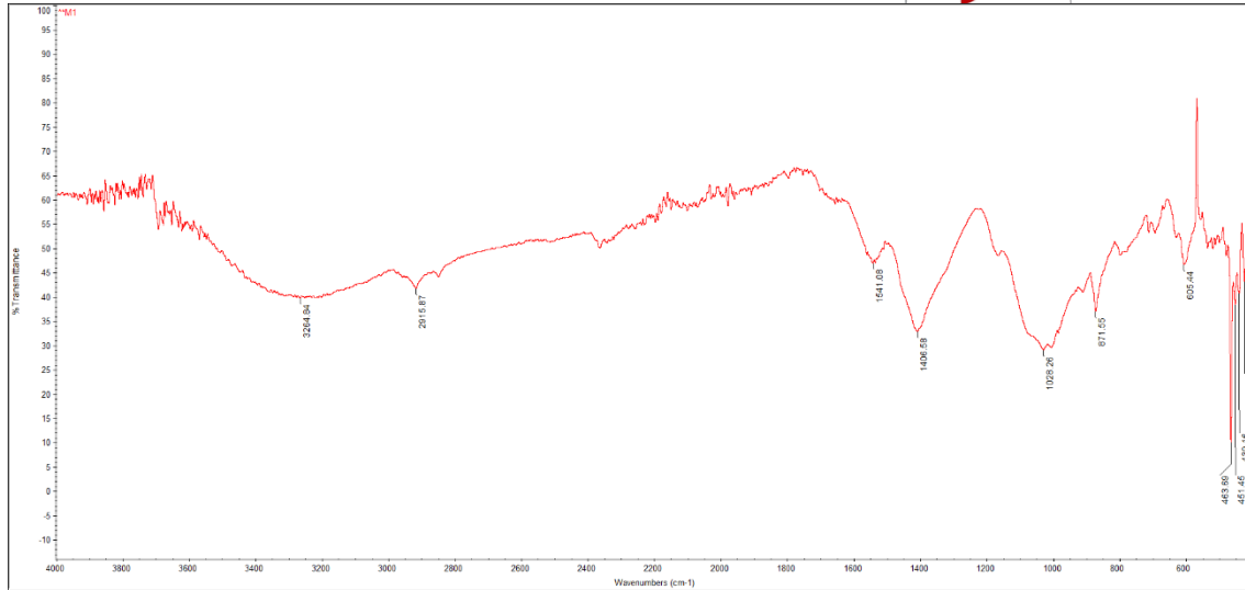
Figura 5. FTIR muestra de perdigón
