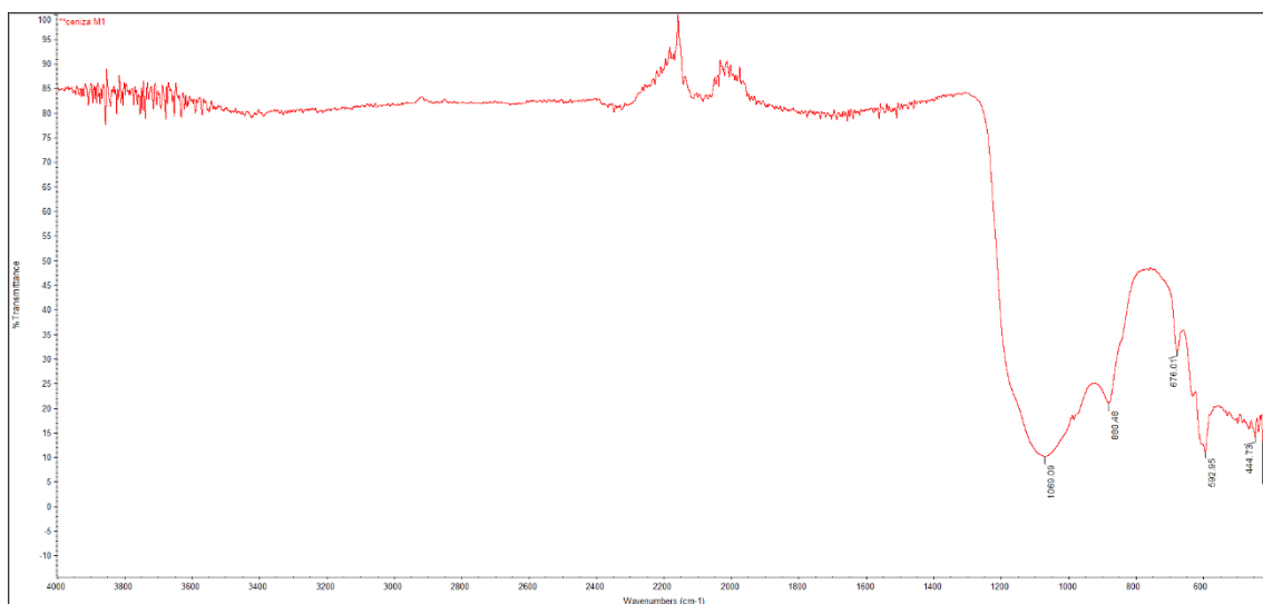
Figura 6. FTIR muestra de ceniza
