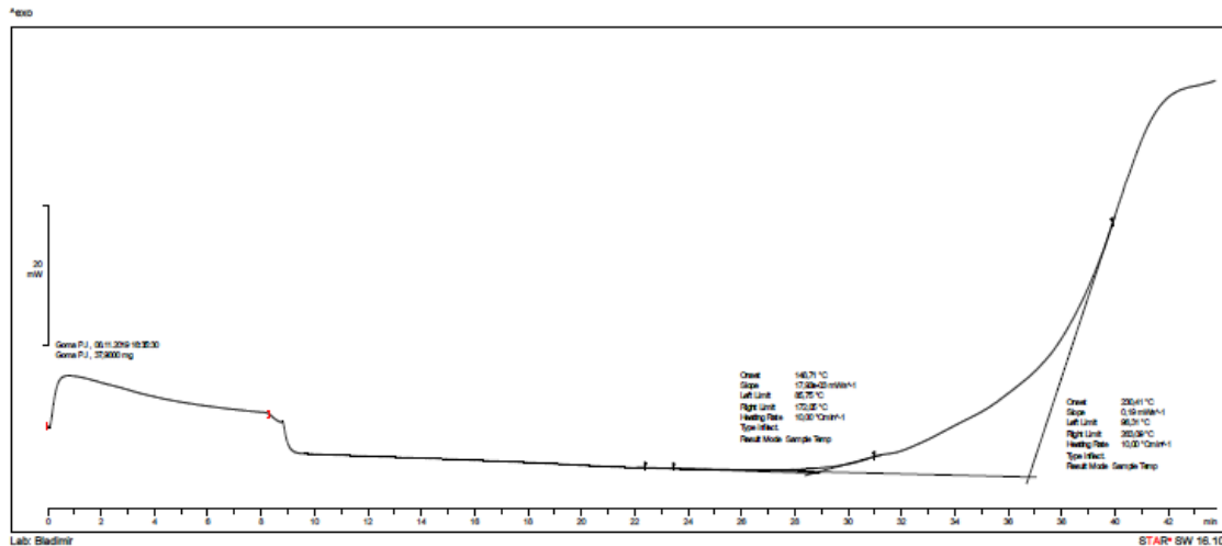
Figura 3. Termograma de -50 °C a 300 °C
